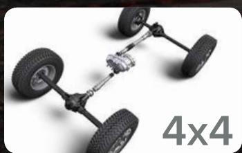
Caja de transferencia Rock-Trac® con ejes DANA 44
